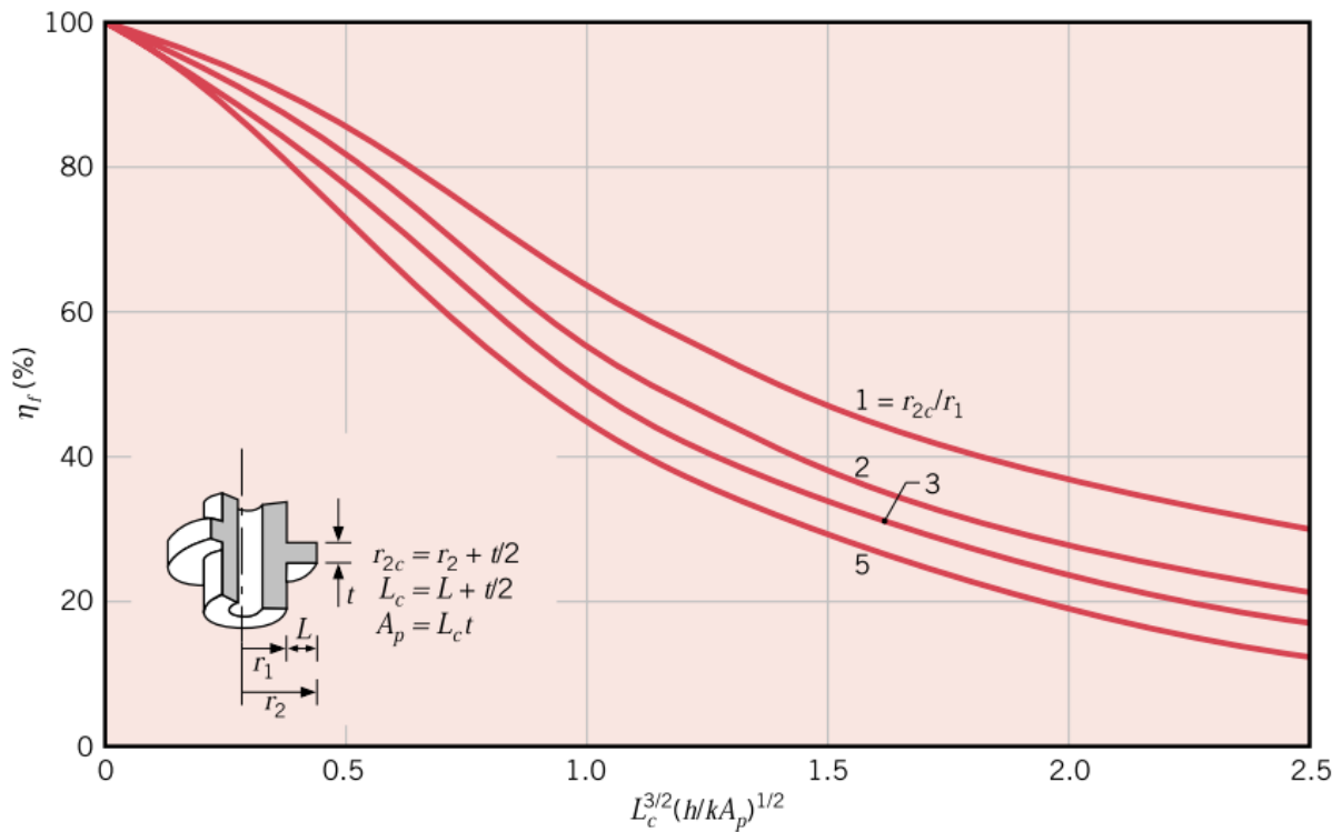
Şekil 2. Dikdörtgen profilli dairesel kanatların verimleri
