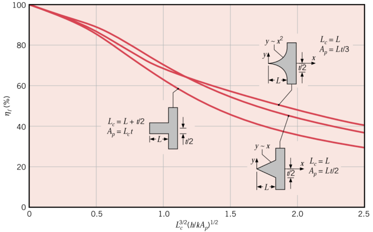
Şekil 1. Dikdörtgen, parabolik ve üçgen profilli düz kanatların verimleri
